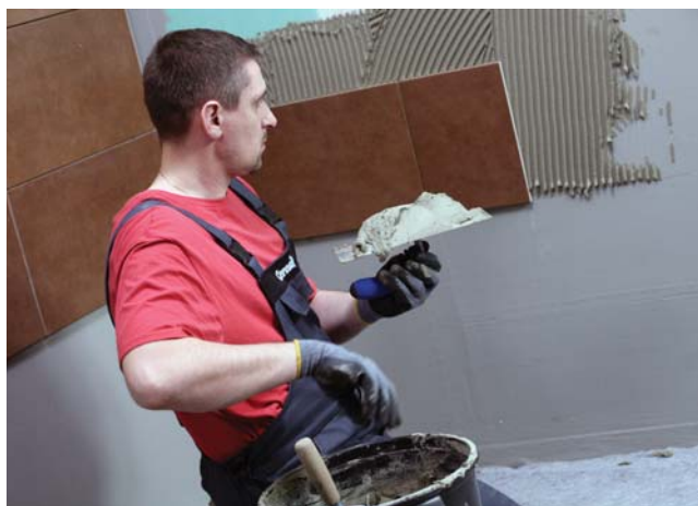
Przy prawidłowo dobranej konsystencji zaprawa zapewnia odpowiednią przyczepność zarówno do narzędzi jak i do podłoża
